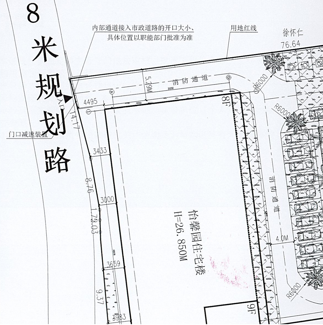
怡馨园住宅楼总平面布置图 1:300
