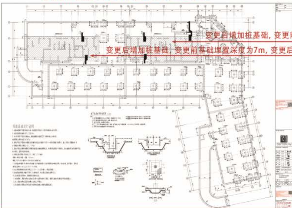
变更前基础布置图
