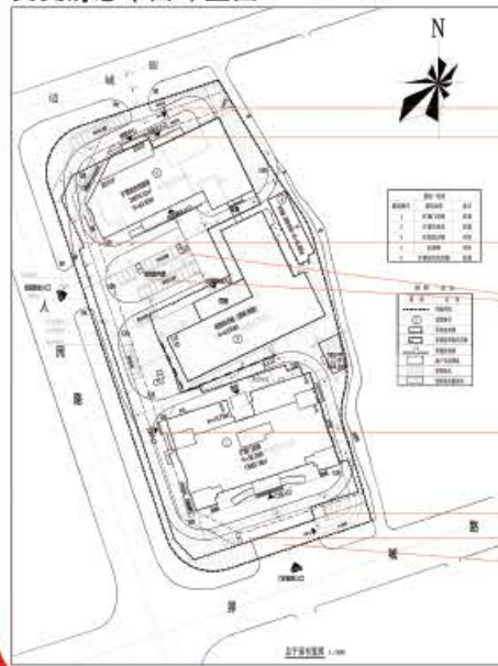
变更前总平面布置图
